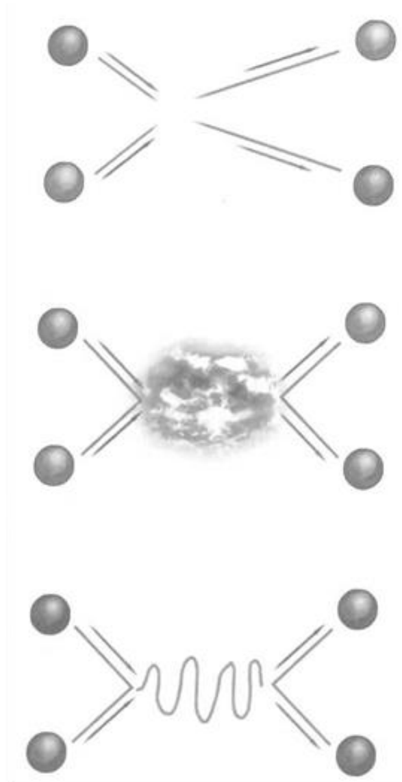
Intercambio de partículas
